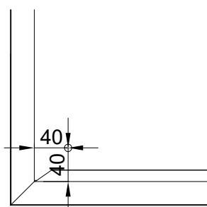
Befestigungspunkt Rückwand
