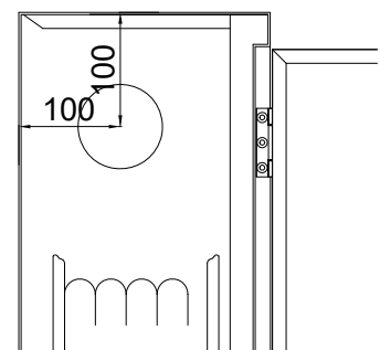
Detail Loch Feuerhahn links/rechts oben
