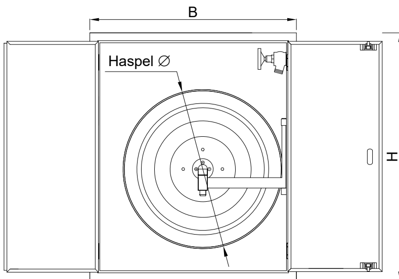
Vorderansicht mit geöffneter Tür
