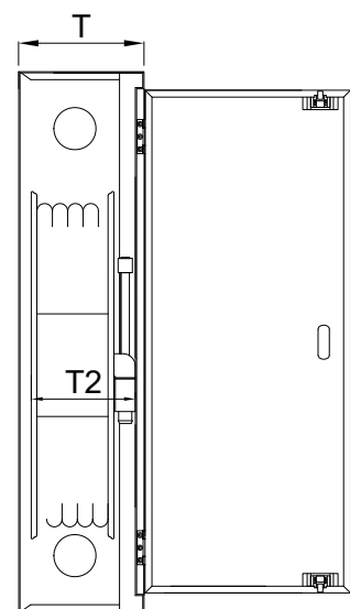
Schnitt Seitenansicht
